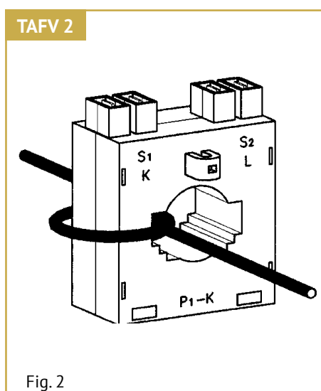
300 / 5A 2 passaggi = 150 / 5A 2 loops = 150 / 5A
