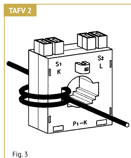
300 / 5A 3 passaggi = 100 / 5A 3 loops = 100 / 5A
